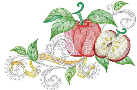
Ape3352c_008.vip
