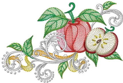
Ape3352a_008.vip
