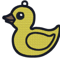
Fsl1771_var_2.vip
