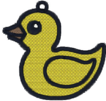
Fsl1771.vip
