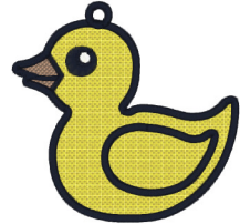
Fsl1771_var_3.vip
