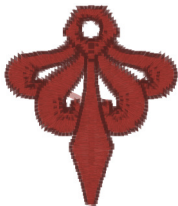
Fsl1310.vip
