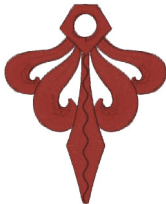
Fsl1310_var_4.vip
