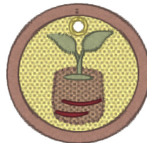
Fsl1407_var_2.vip
