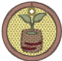
Fsl1407.vip
