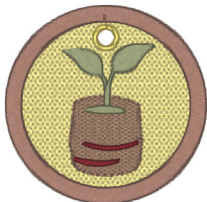
Fsl1407_var_3.vip
