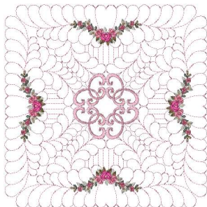
Ape3184a_005.vip
