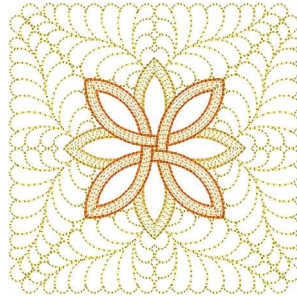
Ape3030b_005.vip
